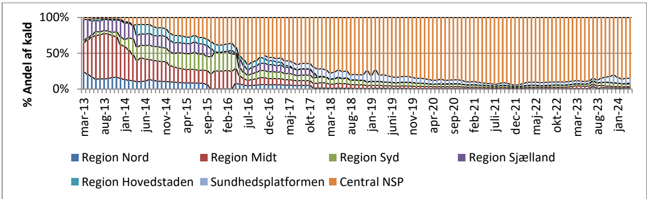
Figur 2: Diagram over fordeling af kald mellem NSP instanser, månedsvise opdeling
