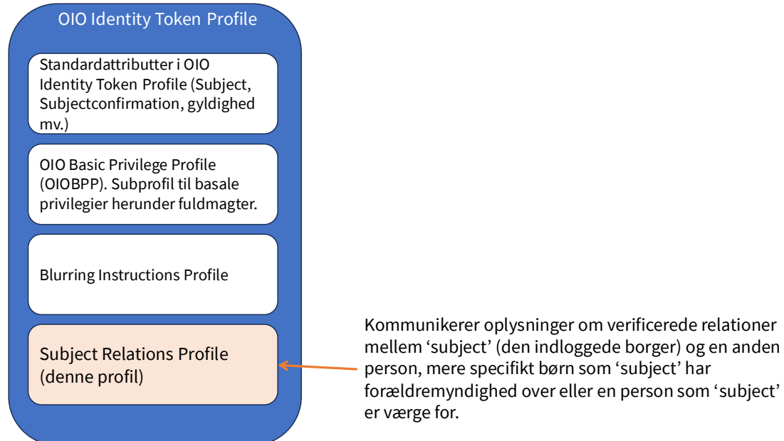
Figur 1: Profilen er en subprofil til OIO Identity Token Profile og har til hensigt at regulere, hvorledes værg- og forældremyndighedsrelationer udtrykkes som SAML attributter.
