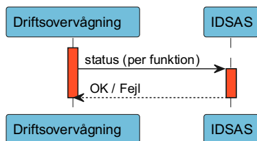
Figur 35: Kontrol af driftsstatus. Driftsovervågningsværktøj kalder periodisk status() på alle IDSAS services for at kontrollere hver enkelt service er kørende.
