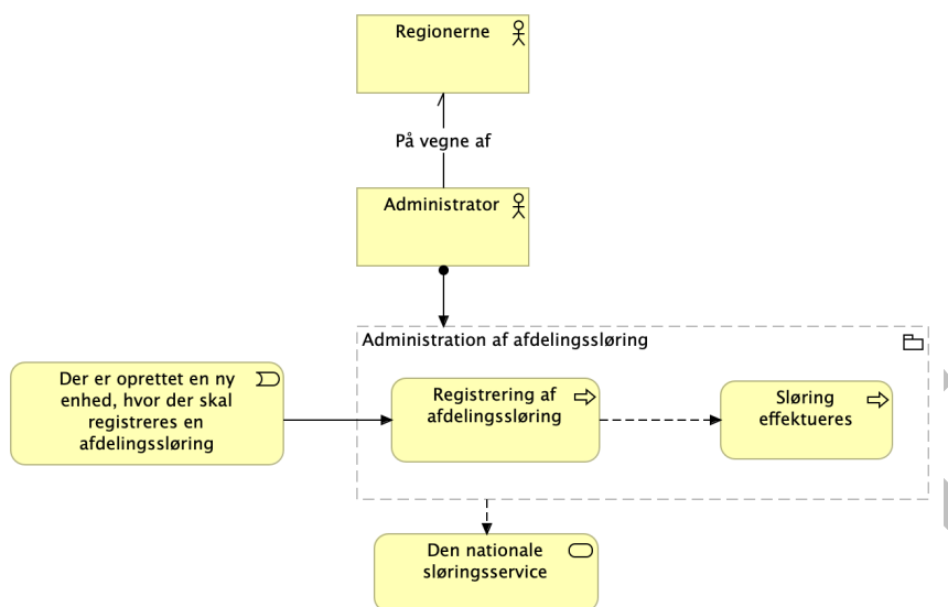
Figur 16: Registrering af en afdelingssløring. Afdelinger angives i SOR klassifikationen, og det kontrolleres, at den angivne SOR-enhed findes ved oprettelse.
