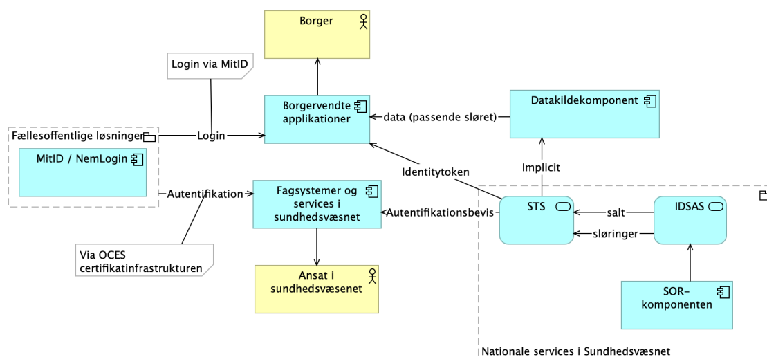
Figur 27 Nationale og fællesoffentlige løsninger der er i spil.
