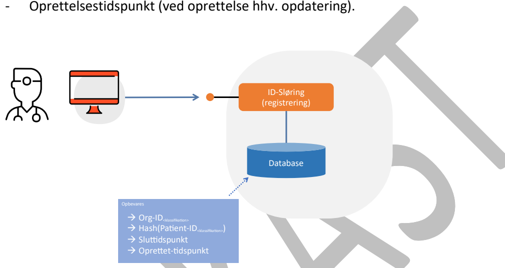
Figur 21: Oplysninger der opbevares per sløringsregistrering.
