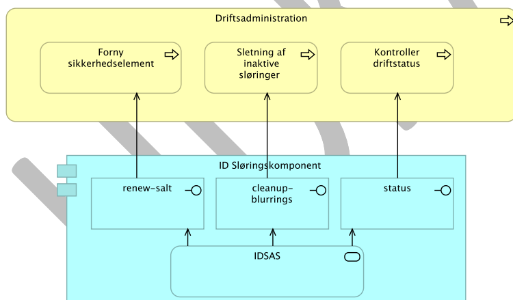
Figur 32 Applikationsunderstøttelse af driftsadministration.
