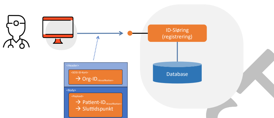
Figur 20: Informationer der medsendes ved registrering af en sløring. Organisations-ID (CVR-nummeret) aflæses fra adgangsbilletten (SOSI ID-kort), patient-ID og sluttidspunkt medsendes som egentlige parametre.
