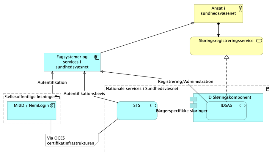
Figur 28: Applikationssammenhæng for registrering og administration af borgerspecifikke sløringer.
