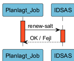
Figur 34: Et andet planlagt job til fornyelse af 'secret salt'.
