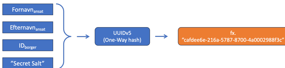
Figur 22: Pseudonymberegningssalgoritmen binder pseudonymer til borgeren og sikret med et "secret salt".
