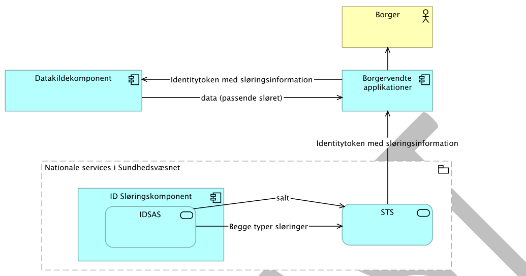
Figur 30: Applikationssammenhæng for effektivering af sløring.
