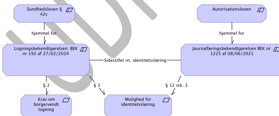
Figur 9: Logningsbekendtgørelsen og journalføringsbekendtgørelsen levner begge mulighed for at ansatte i sundhedsvæsenet kan optræde med anden entydig identitet end navn.
